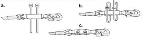
Рис. 2. Фиксация амортизатора стяжками
