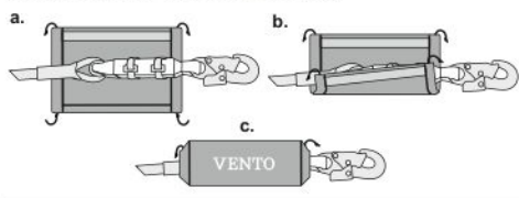
Рис. 3. Установка чехла на амортизатор
