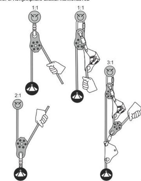
Рис. 3. Популярные схемы полиспастов
